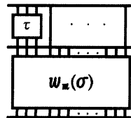
Figure 4: \sigma と \tau の特殊積
