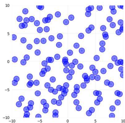
図 1: 連続パーコレーション
