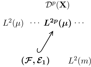
Figure 1: 定理 2.3 (i) の模式図
