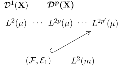
Figure 2: 定理 2.4 (i) の模式図
