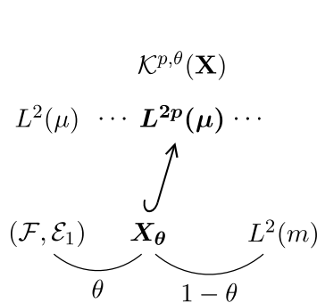
Figure 3: 定理 2.3 (iii) の模式図
