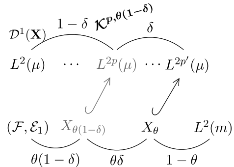
Figure 4: 定理 2.4 (iii) の模式図
