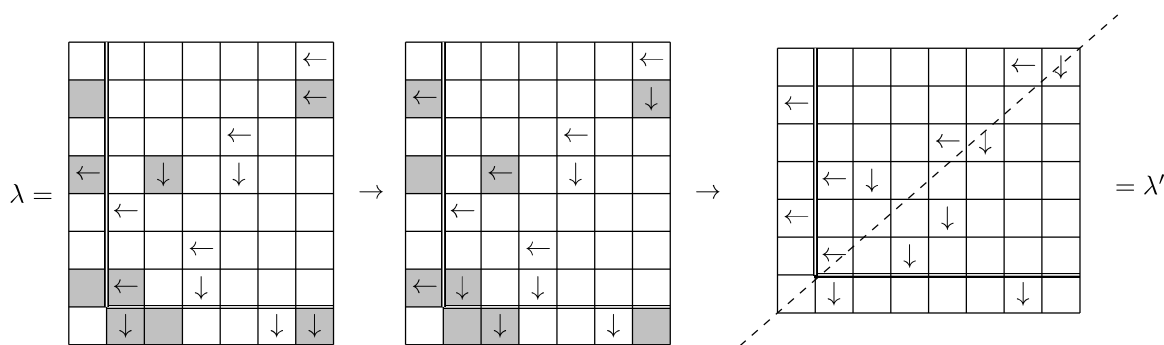
FIGURE 7. (\mathcal{T}_n^k, \text{col}) を用いた対称性 \widehat{\mathcal{B}}_n^k(x) = \widehat{\mathcal{B}}_n^k(x) の説明の例
