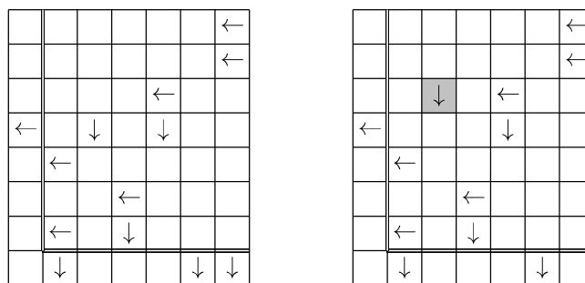
FIGURE 4. サイズ 7 \times 6 の packed alternative tableau
