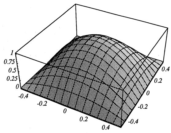
図 7: node が \hat{\Omega}_k の内部にある場合
