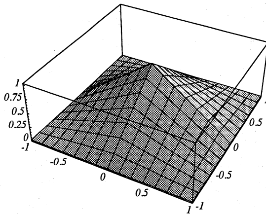
図 4: bi-linear base function
