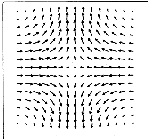
図 15: 流速場 u = (u_1, u_2) (例 2)
