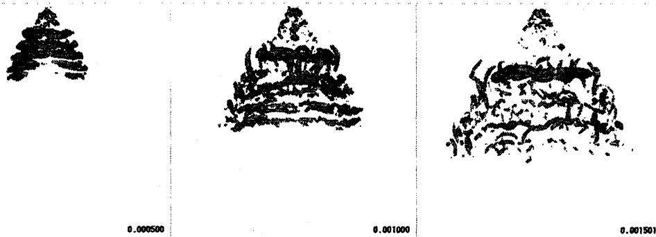
図 11. 渦構造の変化
