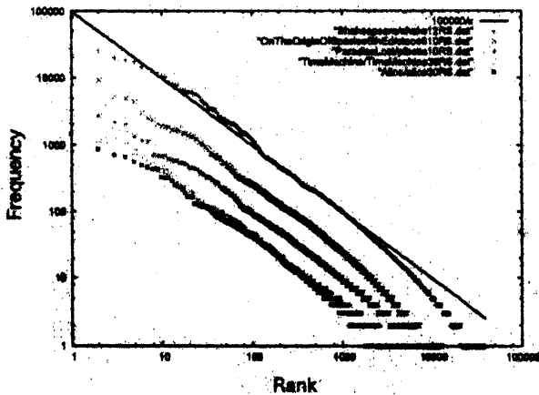
図 2: 書物の単語数に現れる Zipf の法則. 上から, シェイクスピア戯曲集, ダーウィン/種の起原第 6 版, ミルトン/失楽園, ウェルズ/タイムマシン, キャロル/不思議の国のアリス. 直線は \alpha = 1 のフィッティング. 電子書籍データは, Project Gutenberg[9] による.
