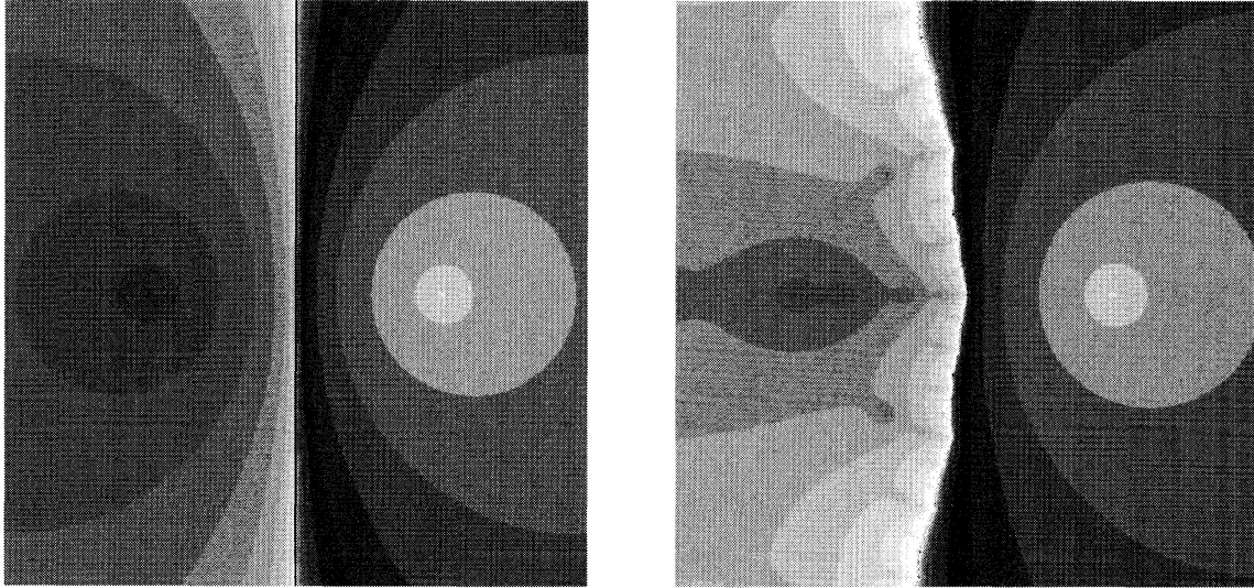
図 1: 左: \lambda = 2 、 \pm 1 は超吸引不動点。 -1 は f の直接特異点。 右: \lambda = 2.2 、 \pm 1 は超吸引不動点、 -1.2 は吸引不動点であり、 f の間接特異点。
