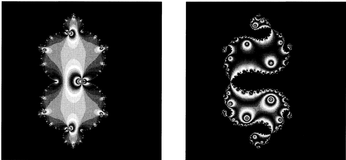
図 3: 左: \varepsilon = 0 右: \varepsilon = 0.1
