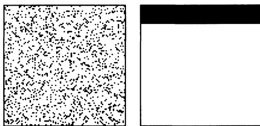
図 6. 時間による空間パターンの変化 ( x_0=0.35, m=0.07, b=0.8 )
