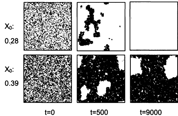
図 5. 時間による空間パターンの変化 (上: x_0=0.28 , 下: x_0=0.39 )
