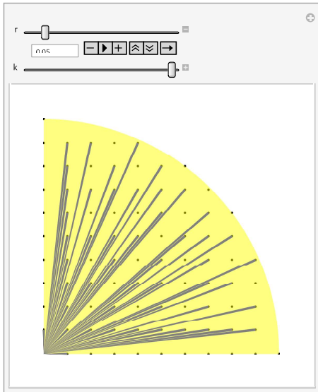
図 1: r < \frac{1}{\sqrt{R^2+1}} のときの果樹園
