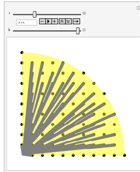
図 2: r > \frac{1}{R} のときの果樹園
