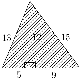
図 1: 組合せて得られる \triangle(13, 14, 15; 84)
