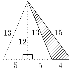
図 2: 除いて得られる \triangle(4, 13, 15; 24)
