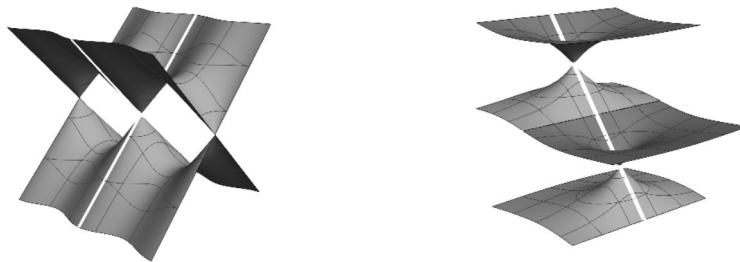
図 2 完備な光的直線を含む極大曲面の例。これらの例は光的直線上に特異点を持っている。
