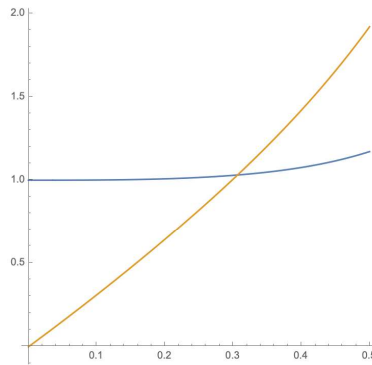
図 4. \lambda \mapsto \Pi_\lambda(\omega) と \lambda \mapsto \Pi_\lambda(\tau) のグラフ
