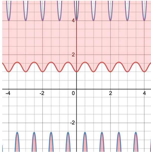
図2 \Delta_2 < 0 となるような (y_2, \epsilon)
