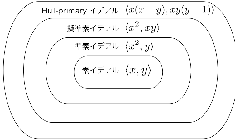
図 5: イデアルの概念の関係
