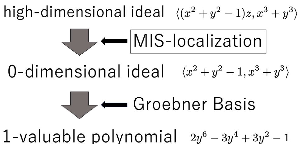
図 4: MIS-localization による 0 次元化
