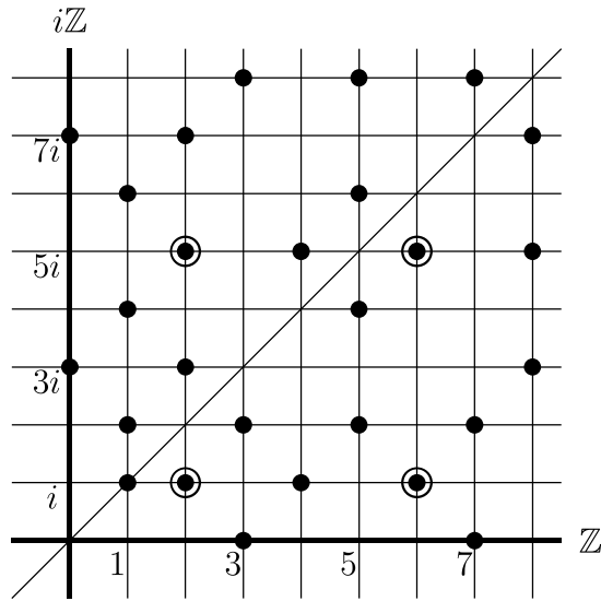
図 1: Gauss 素数でできた正方形
