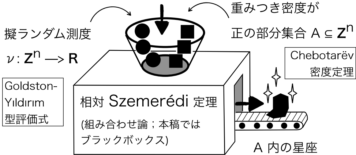
図 2: 証明の 3 大要素
