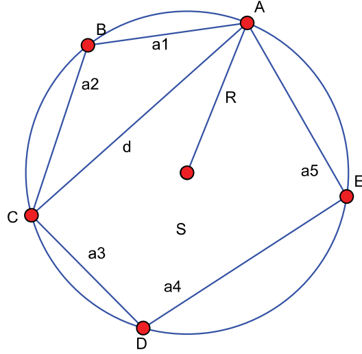
図 1: 円内接五角形問題 (面積 S , 外接円半径 R )
