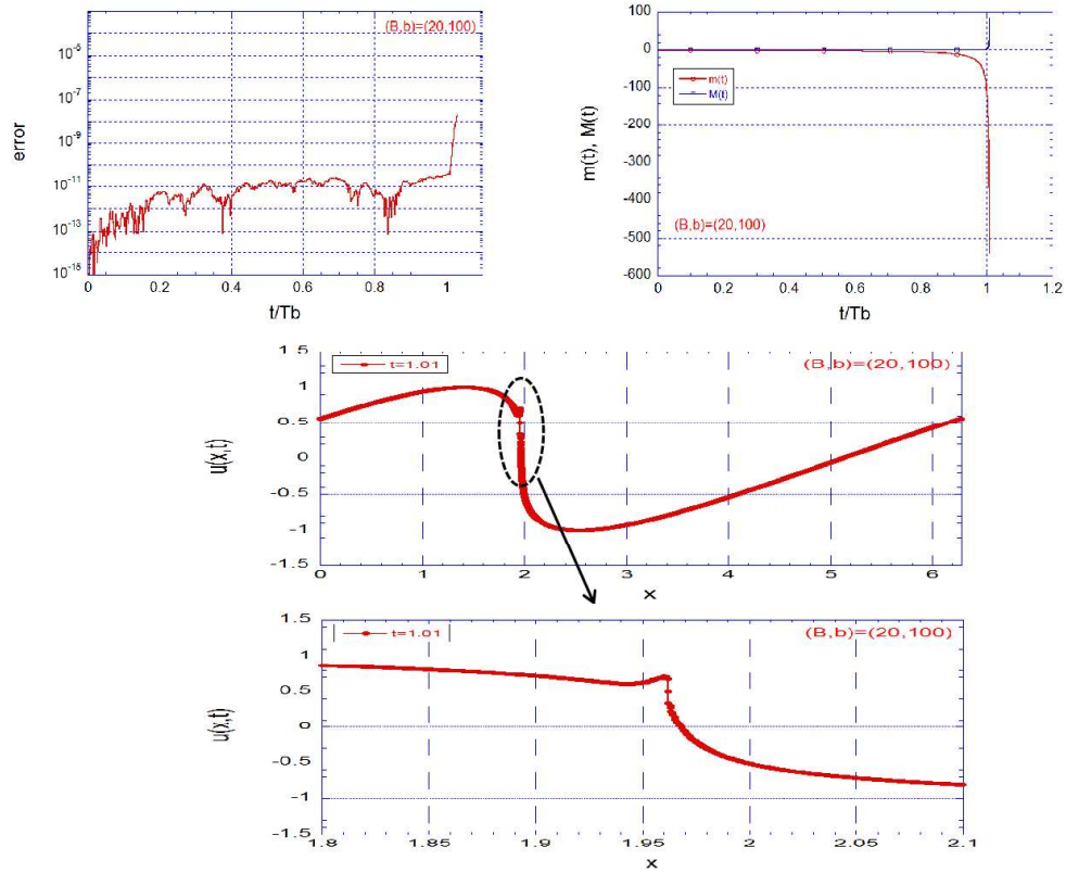
図 7: (B, b) = (20, 100) の場合の結果
