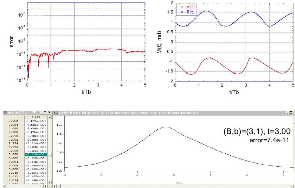
図 2: 砕波が発生しない典型的な計算結果 ( B = 3, b = 1 )
