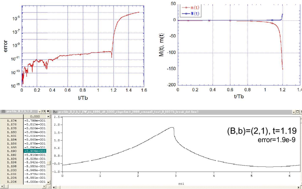
図 1: 砕波が発生する典型的な計算結果 ( B = 2, b = 1 )
