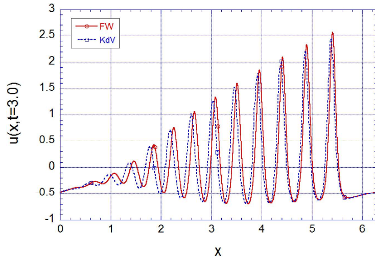
図 7: (B, b) = (20, 100) の場合の結果
