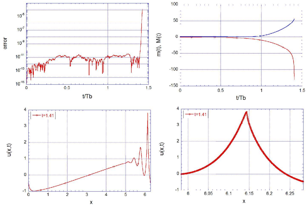
図 4: 「対称的な砕波」の一例 ((B, b) = (50, 30))
