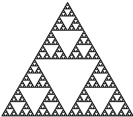
FIGURE 1. Sierpiński gasket
