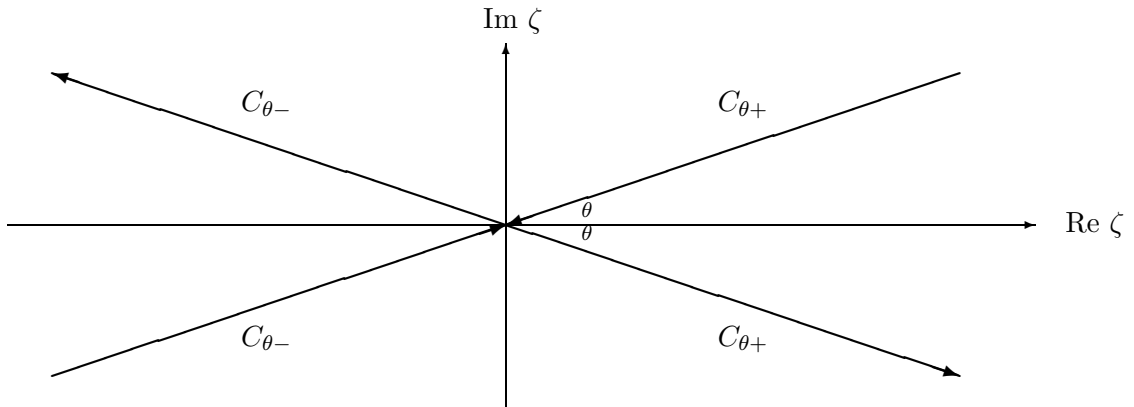
図 4: 積分路 C_{\theta+} ， C_{\theta-}
