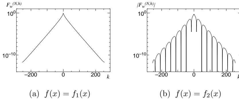
図 5: Fourier 変換の近似結果： F_w^{(N,h)}\left(\frac{2\pi}{Nh}k\right) , N = 512 , h = 0.125
