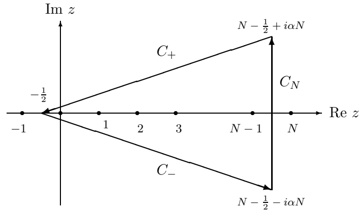
図 2: 積分路 C
