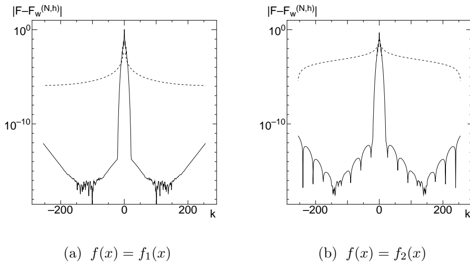
図 7: Fourier 変換の近似誤差 - I_0 -sinh 窓 : F_w^{(N,h)}(\frac{2\pi}{Nh}k) , N = 512 , h = 0.125
