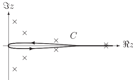
図 2: 積分路 C
