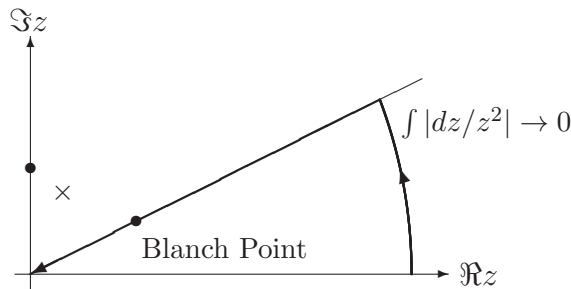
図 5: Contour
