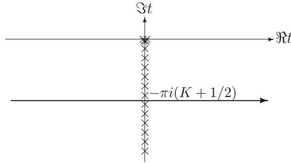
図 4: 積分路
